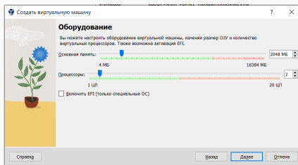
Рис. 2: Настройка оборудования виртуальной машины
